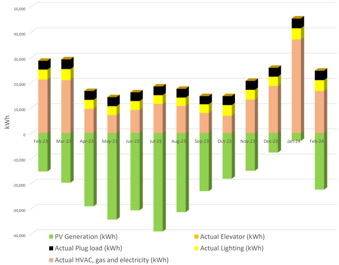
Actual Monthly Compiled (kWh)
