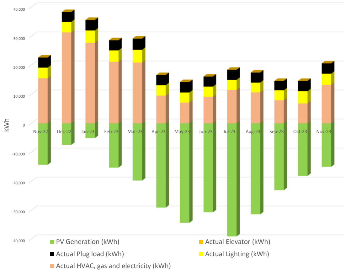
Actual Monthly Compiled (kWh)
