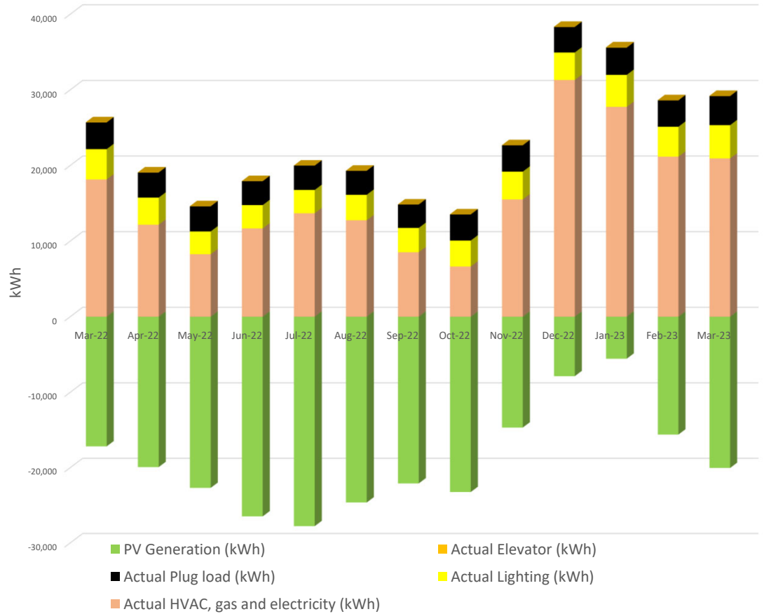
Actual Monthly Compiled (kWh)
